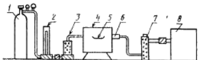
Рисунок 1 — Установка для определения углерода
