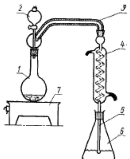
1—дистилляционная колба вместимостью 100 мл; 2—насадка с капельной воронкой; 3—дефлегматор с соединительной трубой; 4—змеевиковый холодильник; 5—барбатор; 6—пробирка-приемник; 7—электролитка.
